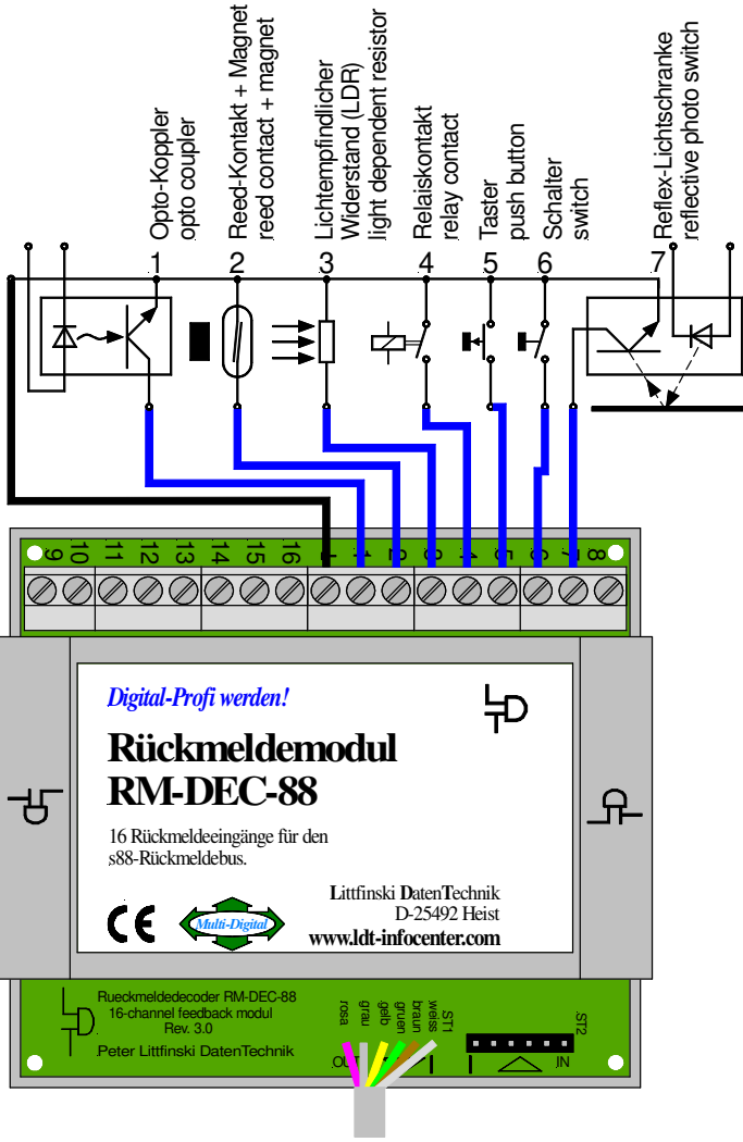
S88- Rückmeldebus S88- feedback bus
