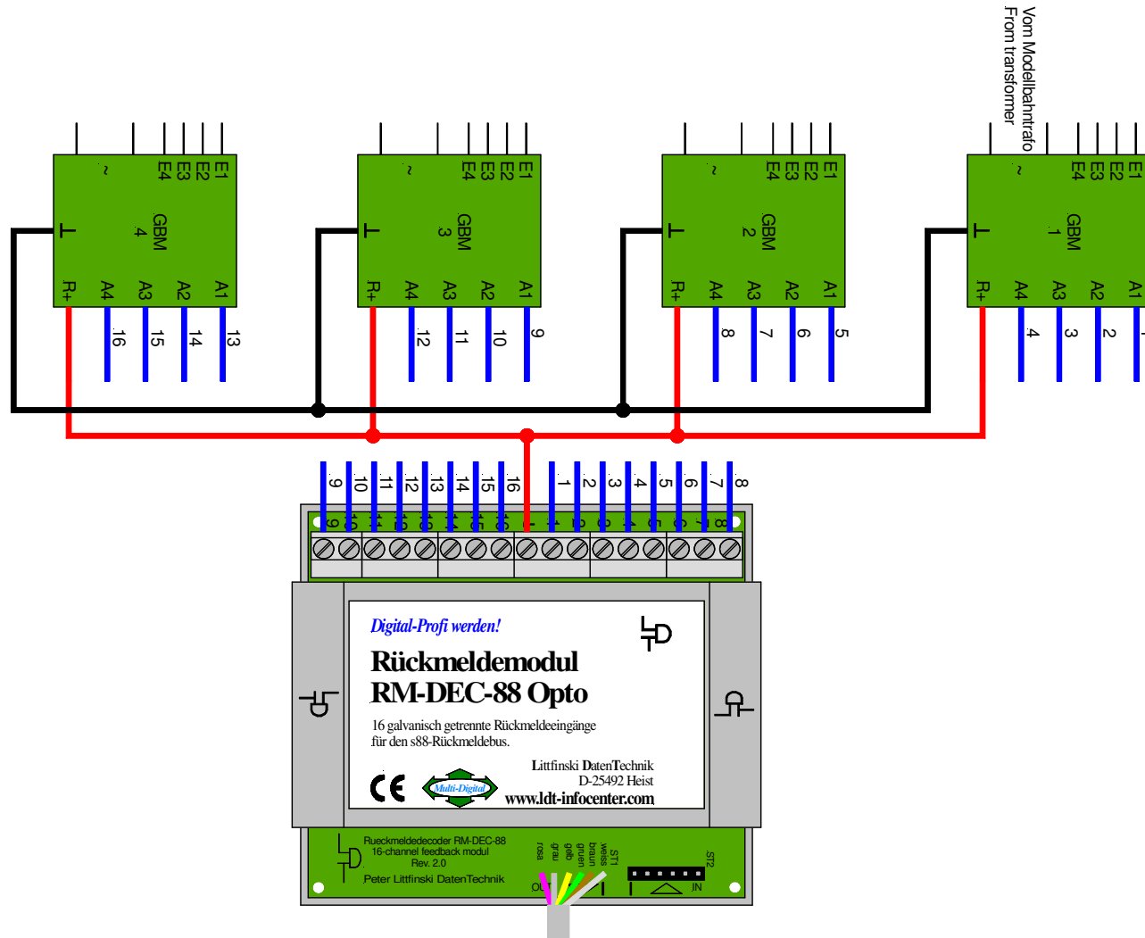
s88- Rückmeldebus s88- feedback bus
