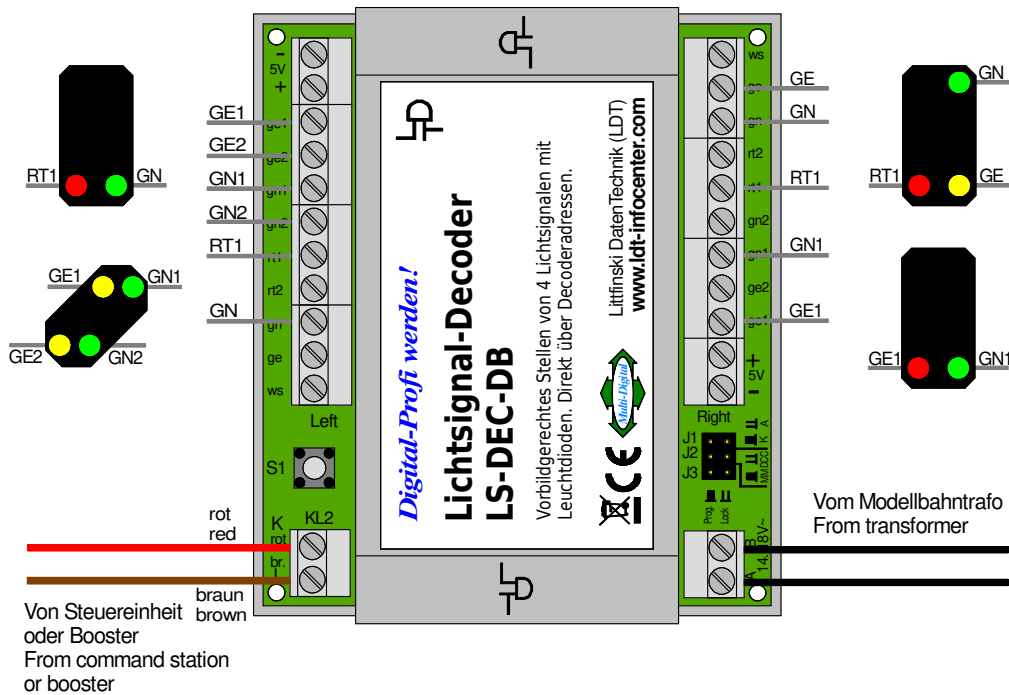
■ Anschlussbeispiel Block- und Einfahrtsignal (page_074)
